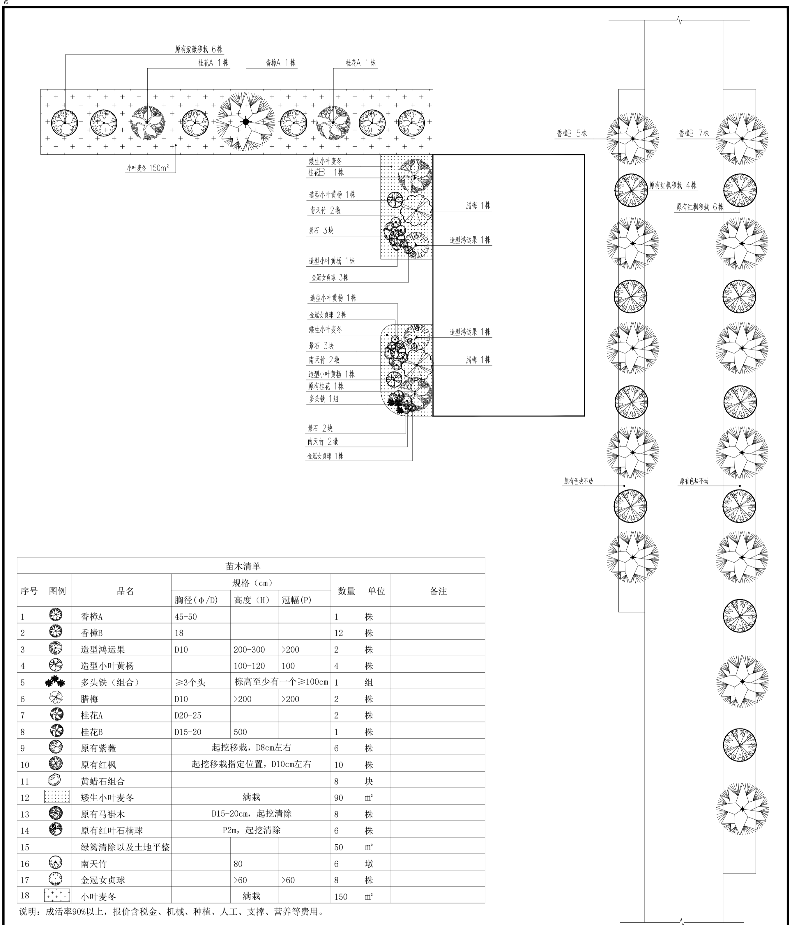
绿化施工图和苗木清单 1:150
